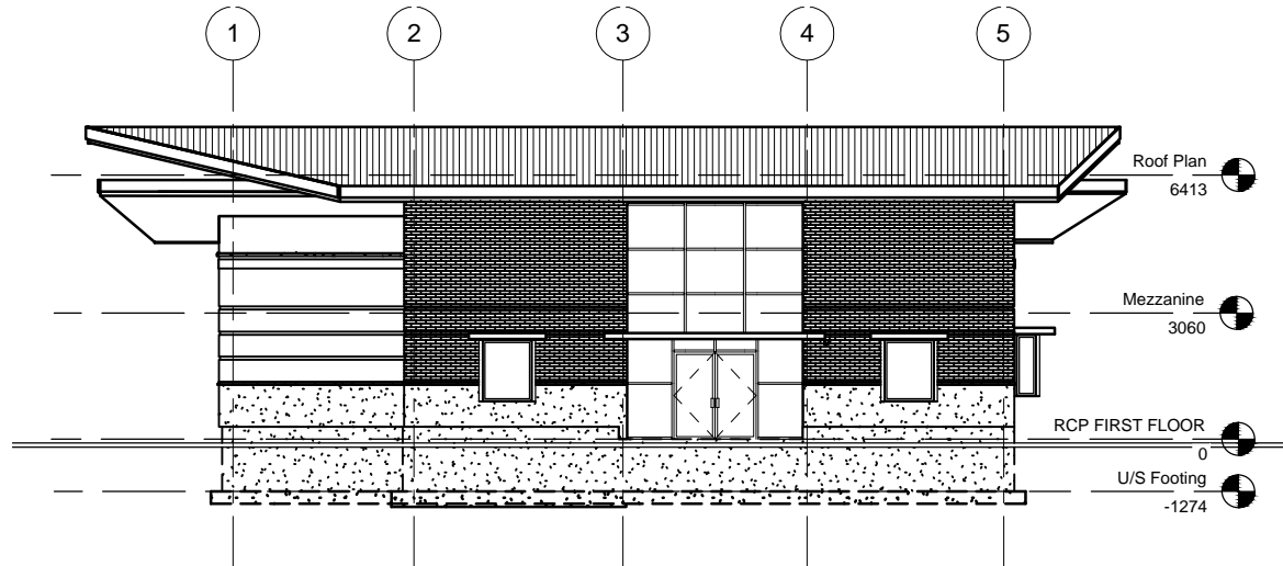
2 South 1 : 100
